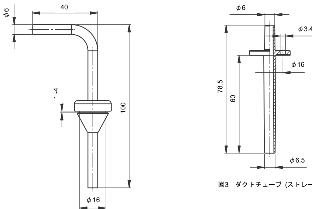
図2 ダクトチューブ (90° タイプ)
