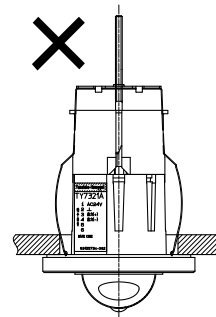
図7 誤った取付例 (両側の足が穴に入った取付)
