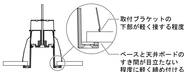
図14 ベースの取付イメージ
