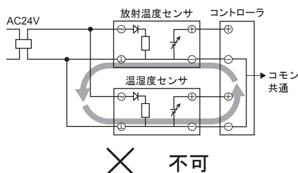
図21 トランス共用
