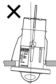
図6 誤った取付例 (傾いた取付)
