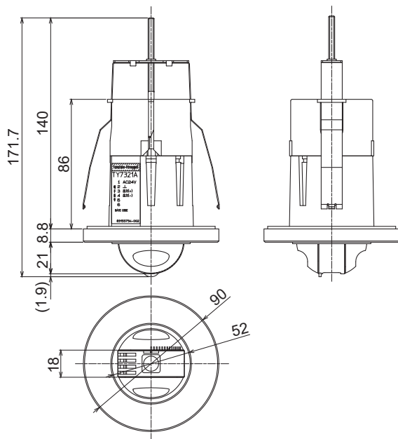
図1 ボックスレスタイプ外形寸法図 (mm)
