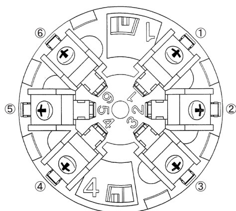
図19 端子図
