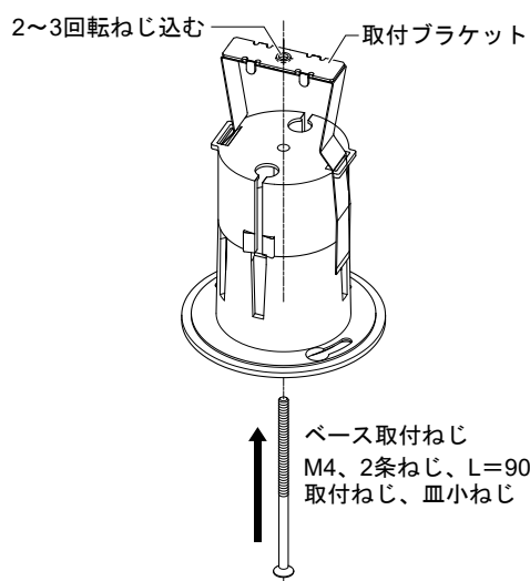
図11 ベース取付ねじの取付ブラケットへの取付
