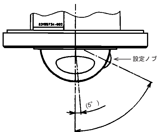
図24 65° 可動
