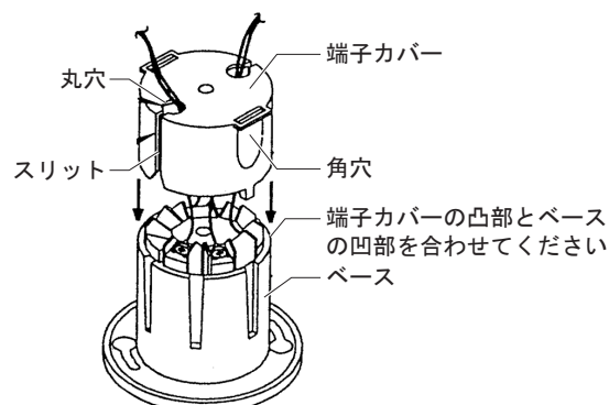
図9 配線方法
