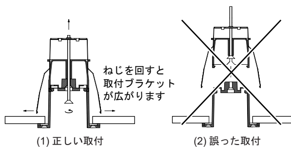
図12 取付穴への設置
