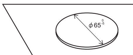
図5 取付穴
