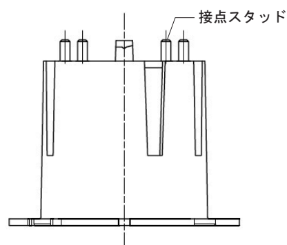
図15 接点スタッドの位置
