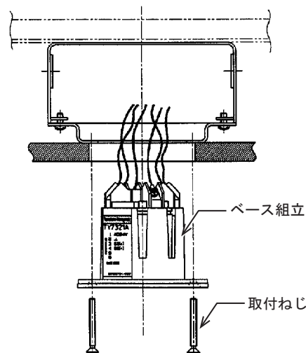
図18 ベースの固定
