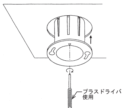
図13 ベースの固定
