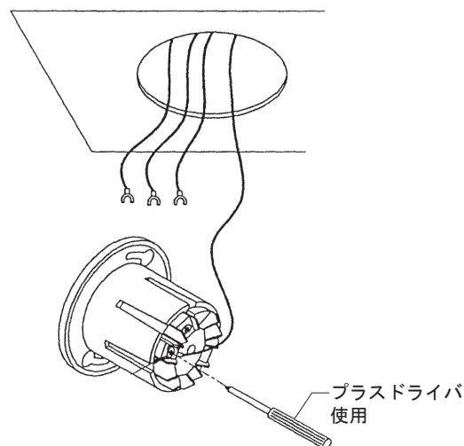
図8 ベースの結線
