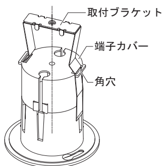
図10 取付ブラケットの組付け
