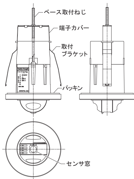
図3 ボックスレスタイプ各部の名称
