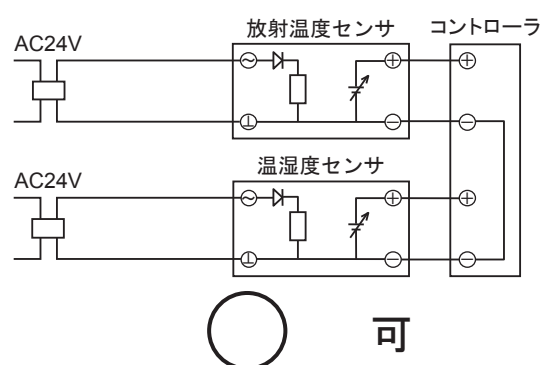
図20 トランス別々
