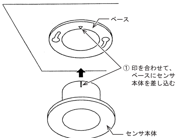
図16 センサ本体の取付け
