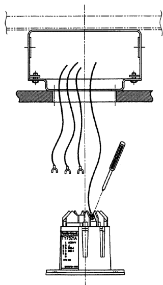
図17 ベースの結線
