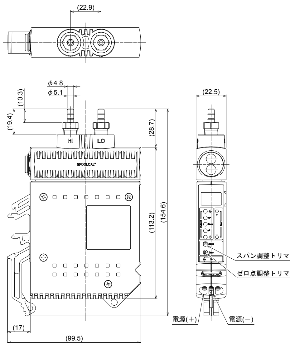
図1 外形寸法図 (mm)
