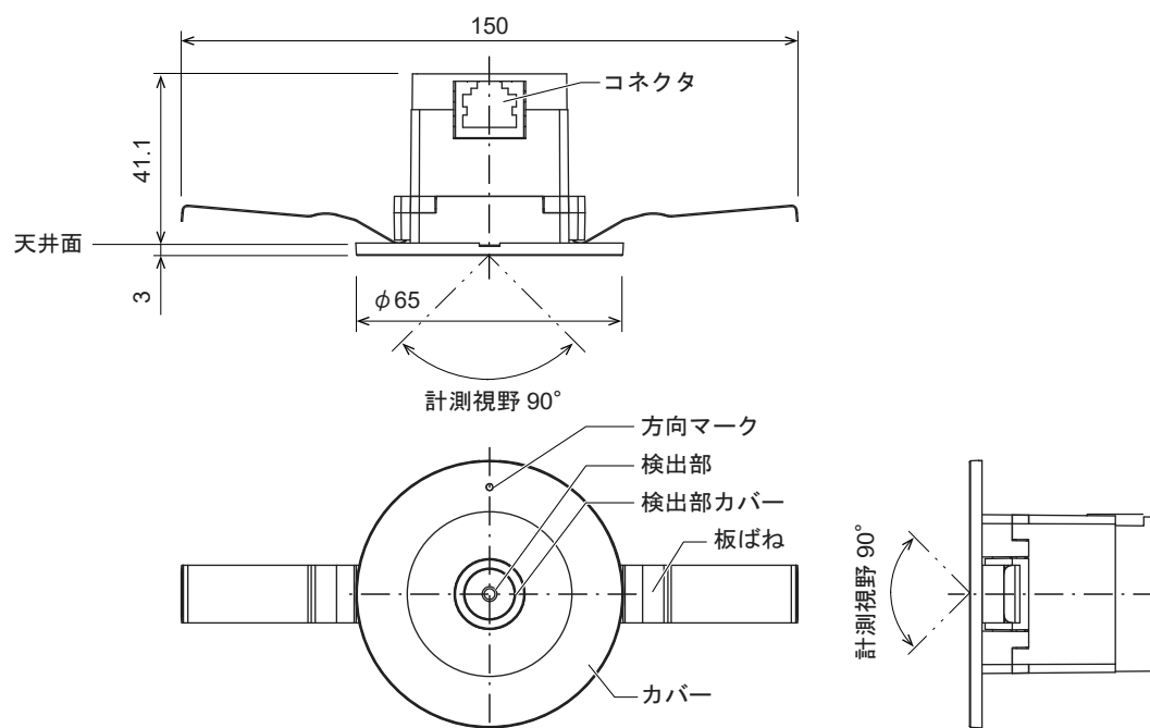
図2 外形寸法図 (mm)
