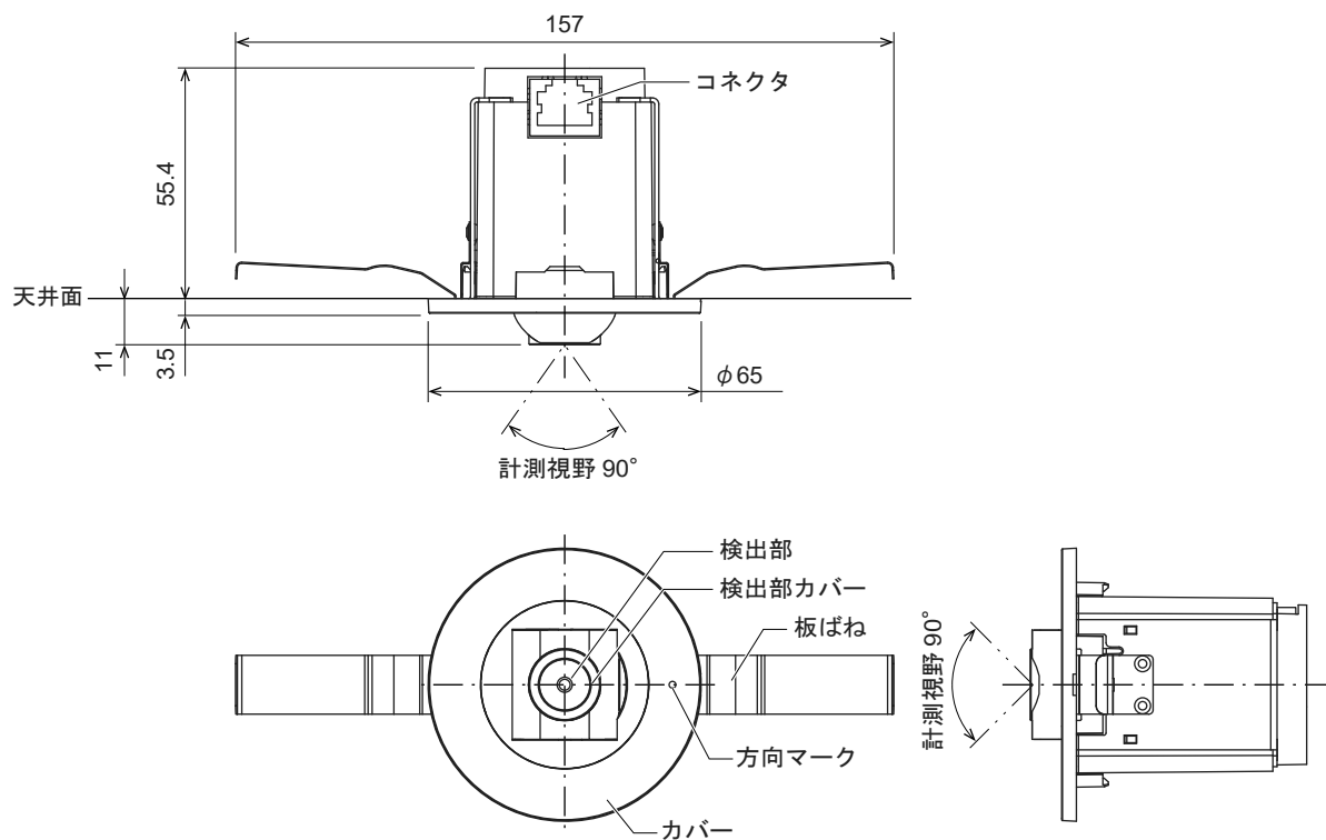
図3 外形寸法図 (mm)
