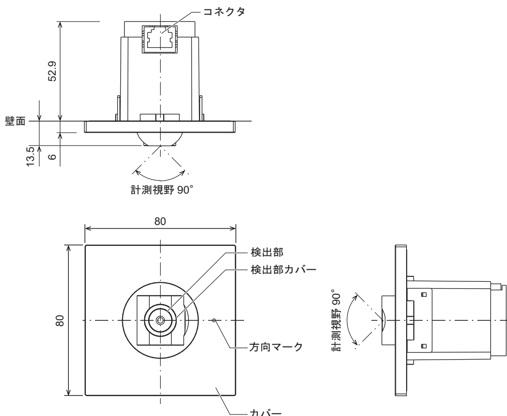
図4 外形寸法図 (mm)
