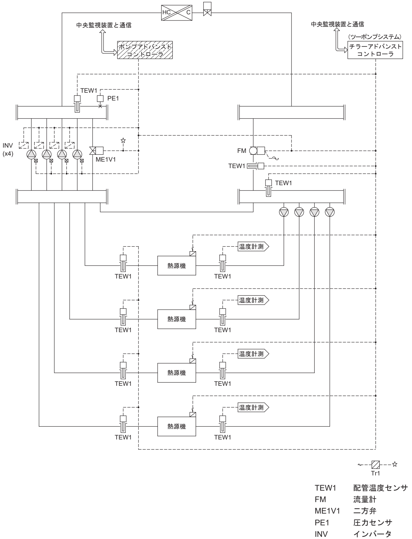
図4 クローズ系ツープンプシステム計装例
