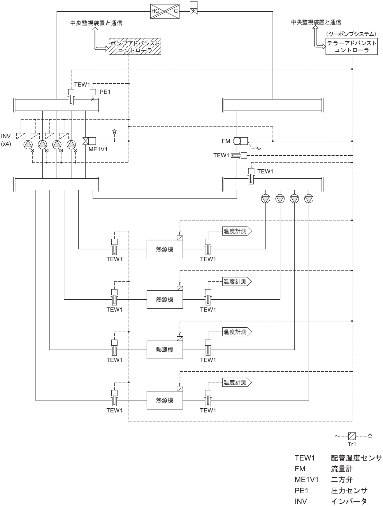
図5 クローズ系ツープンプシステム計装例
