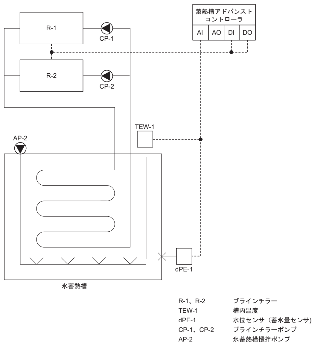
図5 氷蓄熱システム計装例
