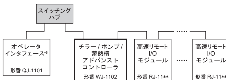
図1 システム構成例
