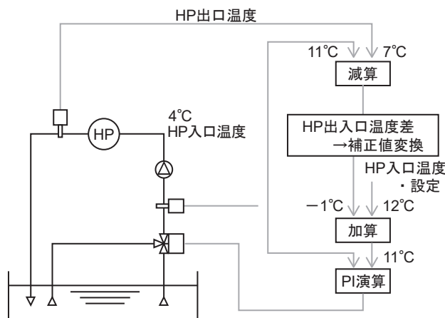
図8 三方弁制御
