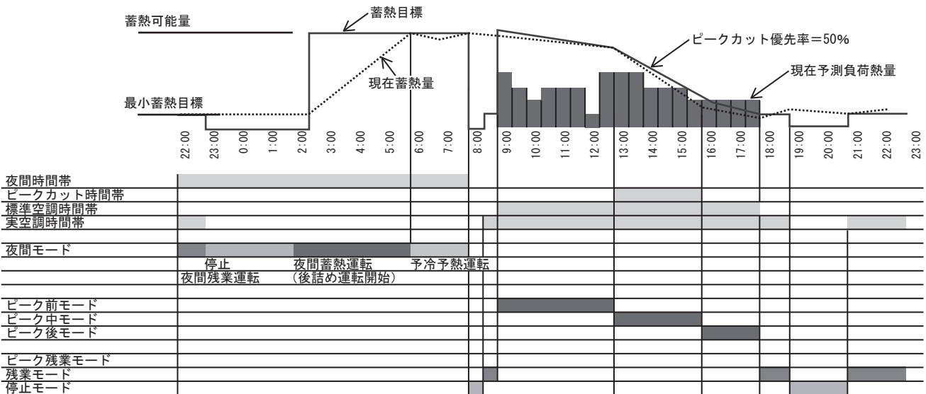
図7 日負荷が大きい例
