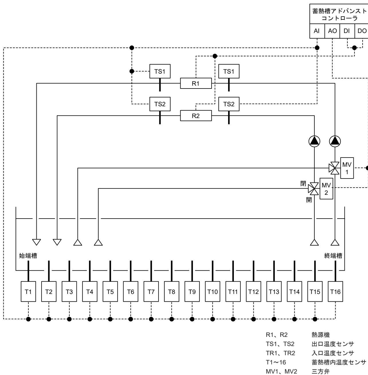
図4 水蓄熱システム計装例
