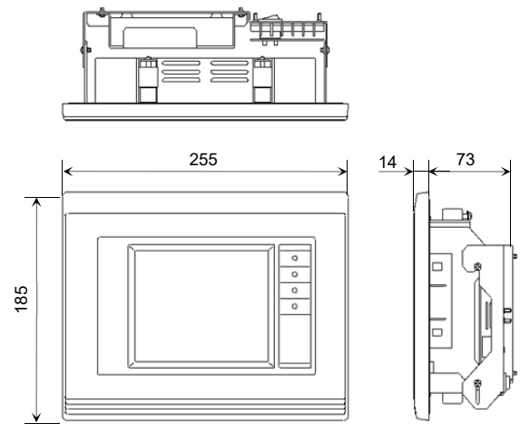
図4 壁埋め込みタイプ(ISDN接続タイプ/LAN接続タイプ共通) (mm)
