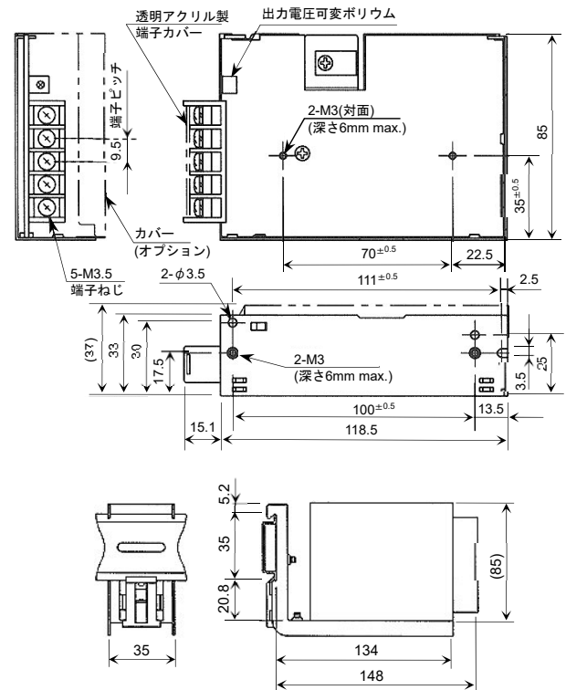
図8 電源ユニット (mm)
