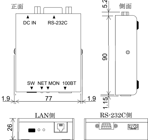
図7 遠隔管理ユニット単体(Web Adapter)(mm)
