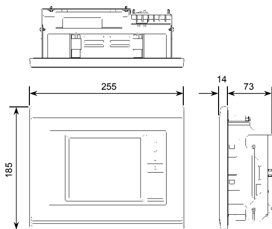
図4 壁埋め込みタイプ (ISDN接続タイプ/LAN接続タイプ共通)
