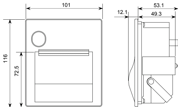
図5 プリンタ単体タイプ
