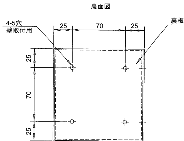
外形図 (mm)
