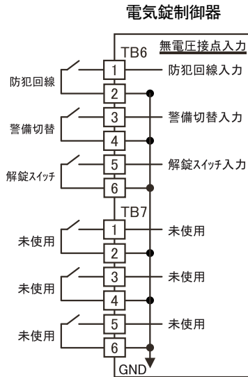
外部信号などとの結線
