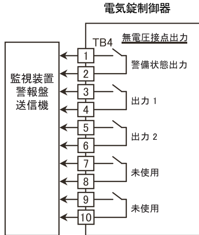
監視装置などとの接続
