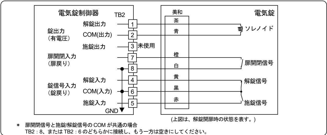
通電時解錠型
