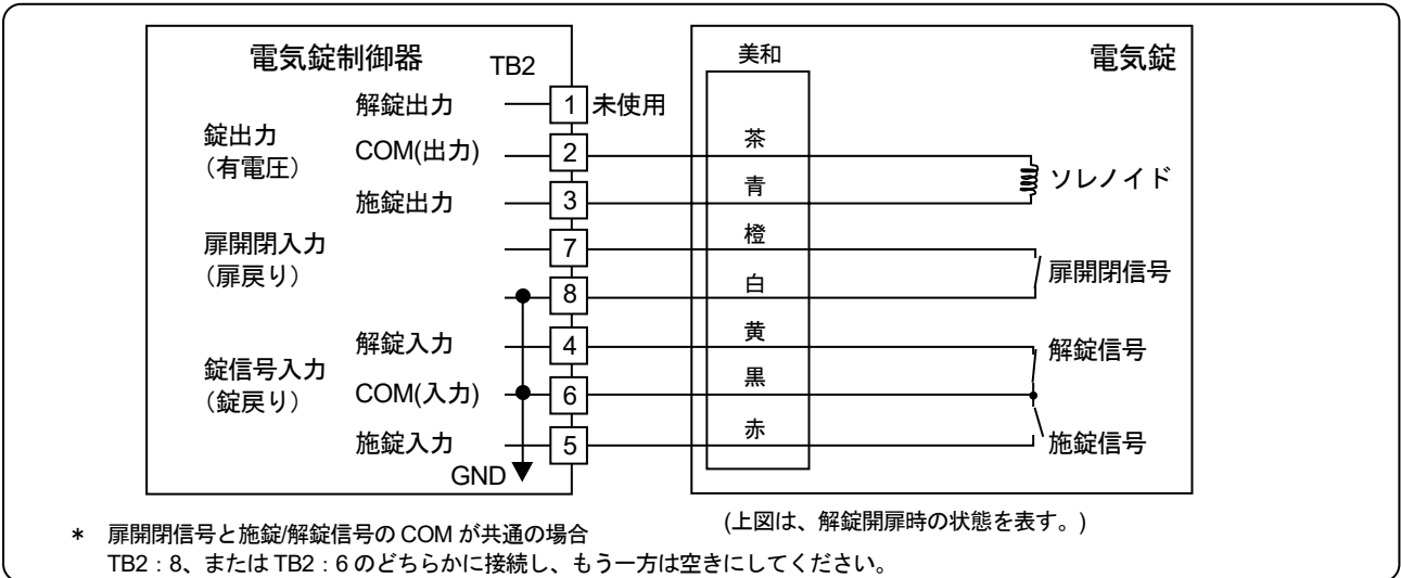
通電時施錠型
