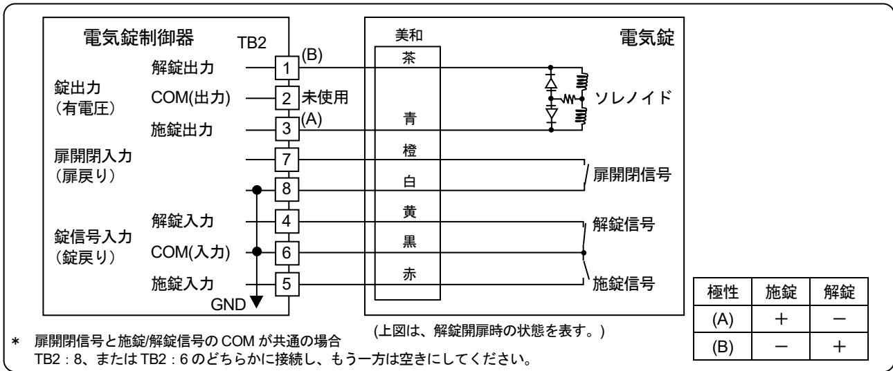
瞬時通電施錠型(2極)
