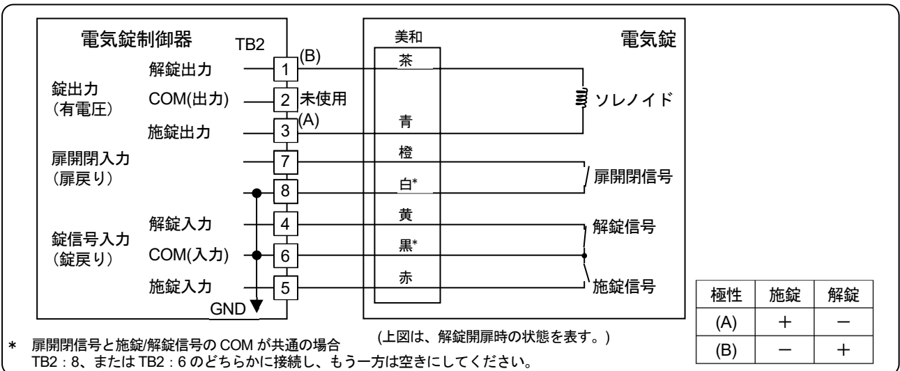
瞬時通電施解錠型(1極)
