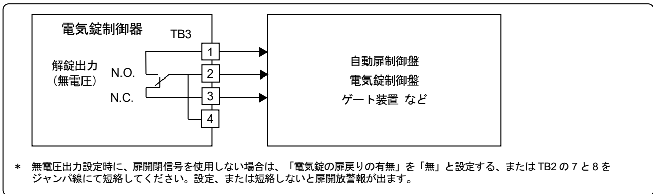
無電圧接点出力先機器
