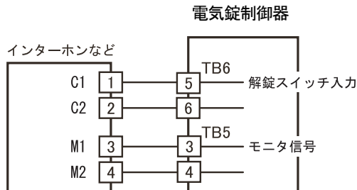
HA端子対応機器との結線
