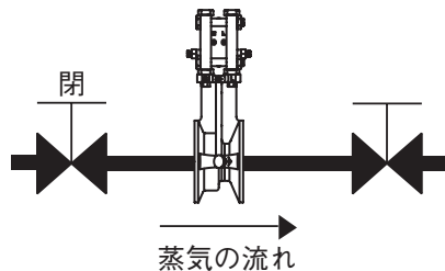
蒸気停止時は一次側バルブを閉とする
