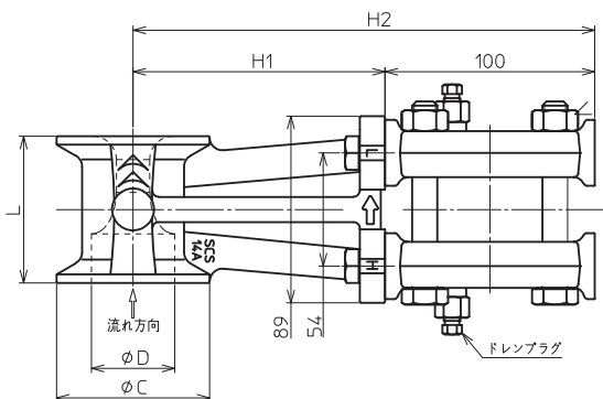
垂直配管取付下から上 (形番：C)
