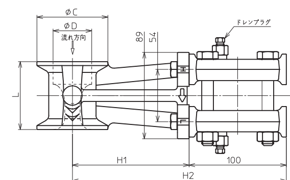
垂直配管取付上から下 (形番：D)
