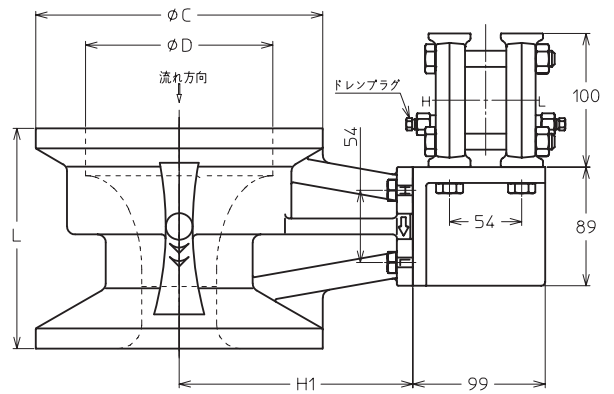
垂直配管取付上から下 (仕様：D)
