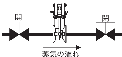
一次側バルブは開／二次側バルブは閉の操作
