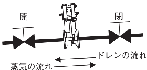
配管勾配が蒸気の流れ方向と逆の場合
