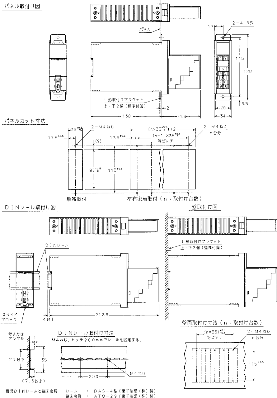
図.3 取付け方法
