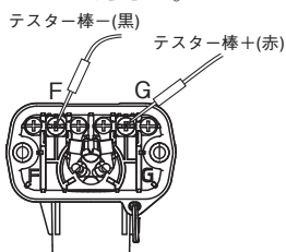
AUD110Cの端子台
